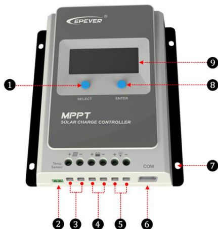
图 1 产品外观
