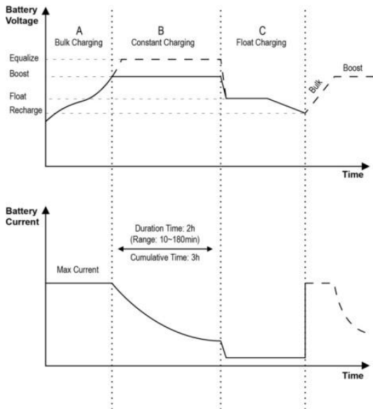
图 1-4 蓄电池充电阶段示意
