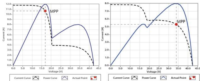
图 1-3 最大功率点跟踪双峰图
