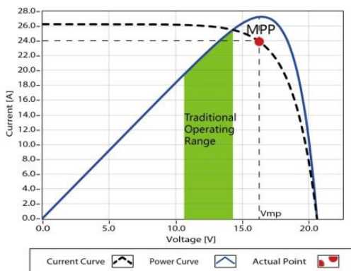
图 1-2 最大功率点跟踪曲线
