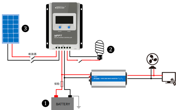
图 2-2 接线示意图
