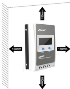
图2-1 安装示意图
