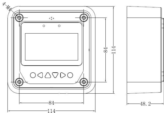
MT52 底壳安装尺寸
