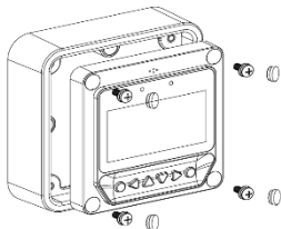
MT52 面板安装
